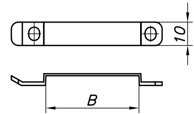
パッチンタイ詳細
