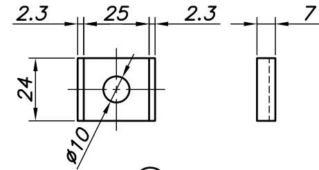
③詳細図
