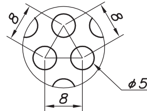
A部詳細
