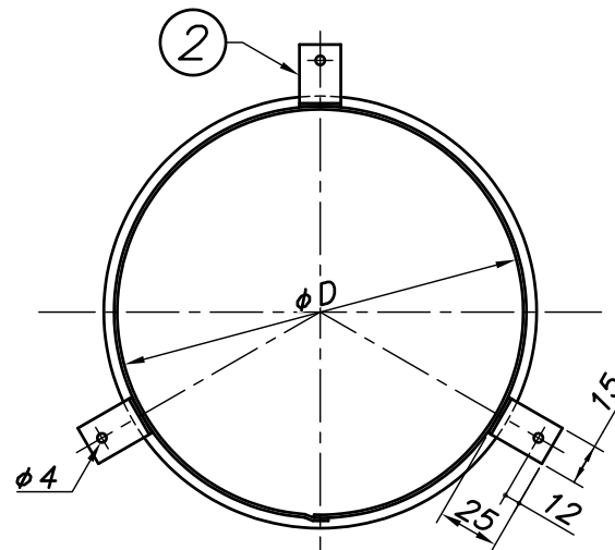
C-C'断面図
