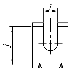
A-A矢視
