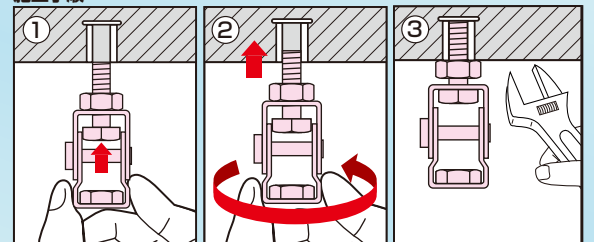
施工手順
